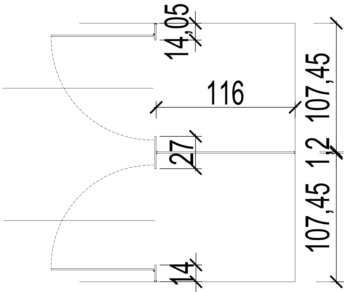
RZUT PRZEGRÓD WC
